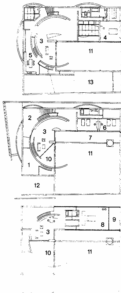
Grundriss von Unter-, Erd- und Obergeschoss: 1 Vorplatz, 2 Halle, 3 Salon, 4 Appartement, 5 Esszimmer, 6 Gästeappartement, 7 Balkon, 8 Appartement, 9 Balkon, 10 Luftraum, 11 Garten, 12 Einfahrt, 13 Garage.
