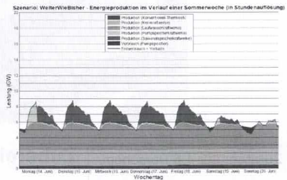
Abbildung 1 Stromerzeugung/-verbrauch während einer Sommerwoche, Szenario „Weiter wie bisher“.
