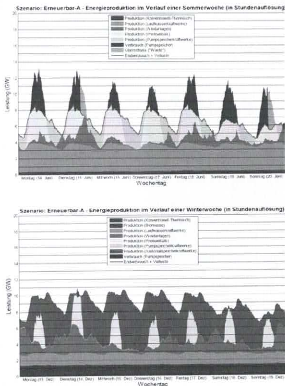
Abbildung 2 Stromerzeugung/-verbrauch während einer Sommer- und Winterwoche mit Mix aus Solar, Wind, Wasser und Biomasse.
